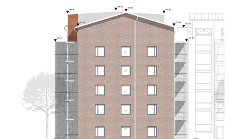
Julkisivu koilliseen
